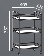
Carro c/ruedas 3 repisas acero cromado 2928
