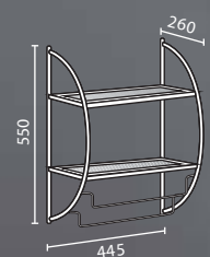
Estantería 2 repisas frente curvo acero niquelado cromado 2924
